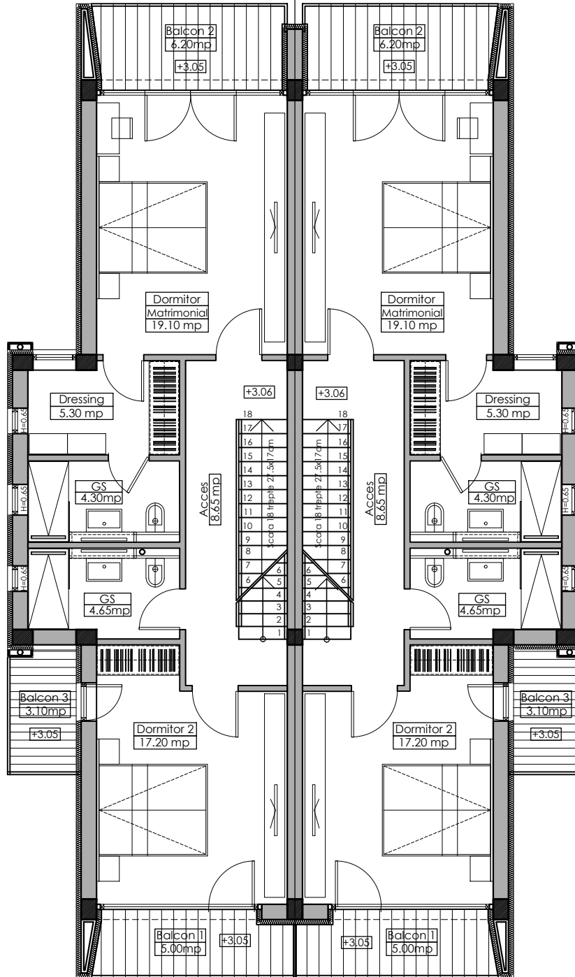
Etaj 1_Poz.4 ÷ 15. Ap: C25-A ÷ C36-A 4 CAMERE
